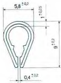
Art. 33.003 Gocciolatoio standard per vetture, colore argento (21) e nero (1) in rotoli da mt. 25.
