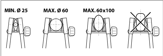
POMELLO ANTIFURTO (DI SERIE) SECURITY KNOB (AVAILABLE)
